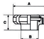
ΦΙΝΙΣΤΡΙΝΙΑ ΔΕΞΑΜΕΝΩΝ ΠΛΗΡΗΣ ΜΕ ΛΕΙΑ ΑΚΡΑ ΓΙΑ ΣΥΓΚΟΛΛΗΣΗ D.400
