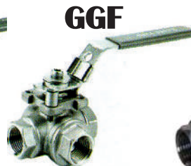
ΣΦΑΙΡΙΚΟΣ ΚΡΟΥΝΟΣ BSP INOX 316 FB 1000 LBS ΤΡΙΣΤΟΜΟΙ
