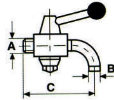
ΚΑΝΟΥΛΑ ΚΩΝΙΚΗ ΚΥΡΤΗ ΒΟΛΤΑΣ 304 G. 966
