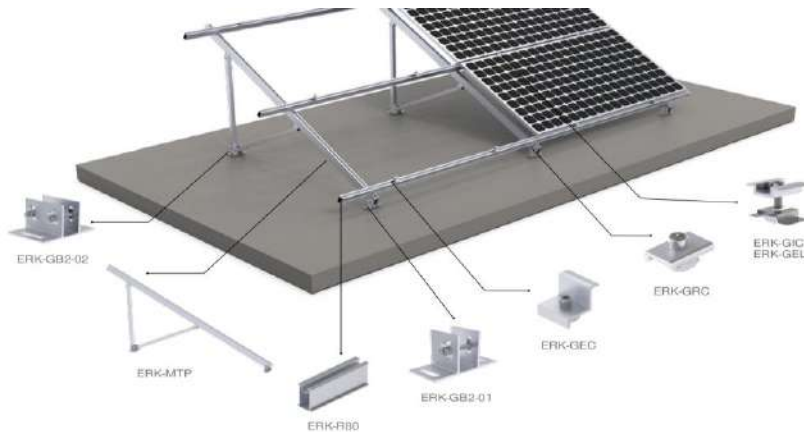
Σύστημα Στήριξης Φ/Β πλασίων σε επίπεδες Οροφές
