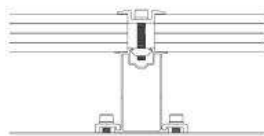
ΣΦΙΓΚΤΗΡΑΣ ΓΙΑ ΠΡΟΦΙΛ R80S ΣΕΤ GRC-35
