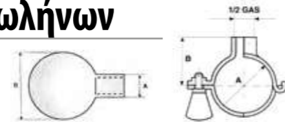
ΣΤΗΡΙΓΜΑΤΑ ΣΩΛΗΝΩΝ
