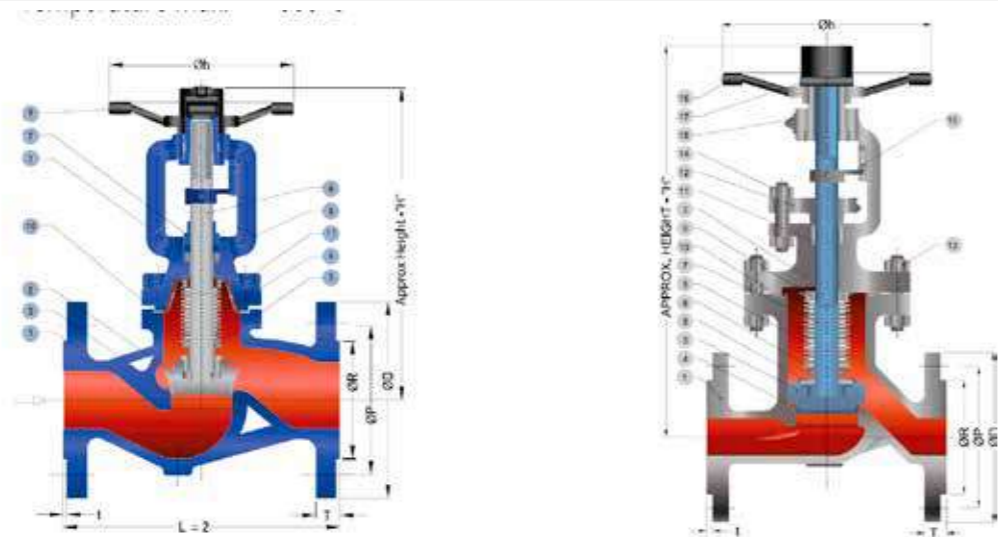
ΑΤΜΟΦΡΑΚΤΗΣ ΦΥΣΟΥΝΑΣ (BELLOW)
