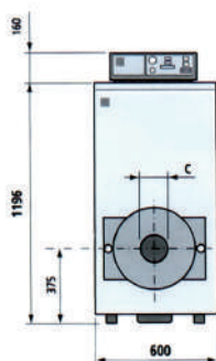
ΕΜΠΡΟΣΘΙΑ ΟΨΗ
