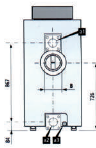
ΠΙΣΩ ΟΨΗ
